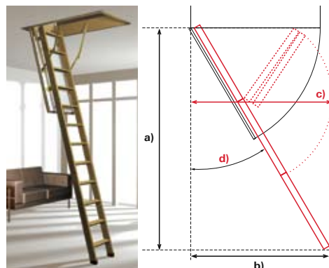
a) чистая высота помещения: от 220 до 286 см b) основание лестницы: от 131 до 87 см c) расстояние, необходимое для разворота лестницы: от 160 до 152 см d) угол: от 22° до 16°
