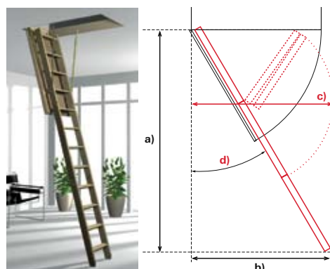
a) чистая высота помещения: от 220 до 285 см b) основание лестницы: от 137 до 88 см c) расстояние, необходимое для разворота лестницы: от 162 до 153 см d) угол: от 22,5° до 16,5°
