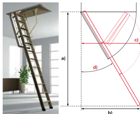
a) чистая высота помещения: от 220 до 287 см b) основание лестницы: от 135 до 87 см c) расстояние, необходимое для разворота лестницы: от 162 до 153 см d) угол: от 22° до 16°
